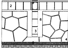
ANCLAJE DE CASTILLO EN MAMPOSTERIA
