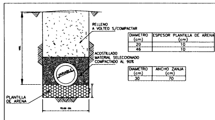
ZANJA TIPO SIN ESCALA
