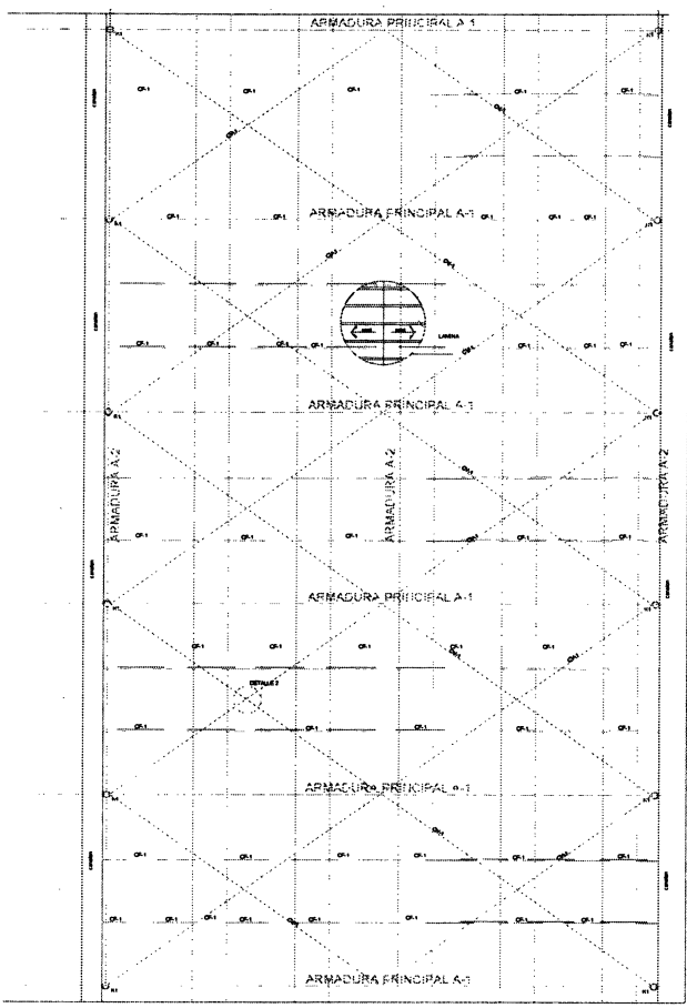
PLANTA ESTRUCTURA METALICA ESCALA 1:10
