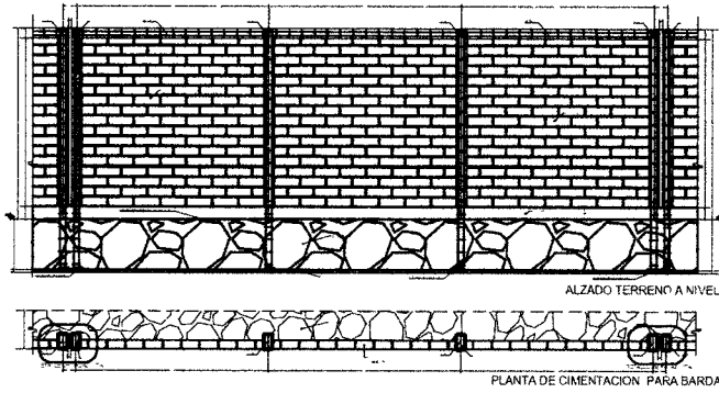
PLANTA DE CIMENTACION PARA BARRA
