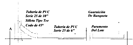
VISTA A-A'
