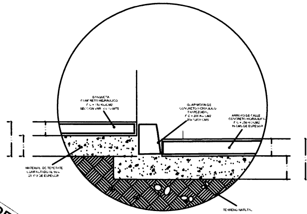
Detalle (C) seccion de banqueta
