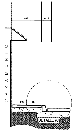
SECCION DE CALLE SIN ESCALA
