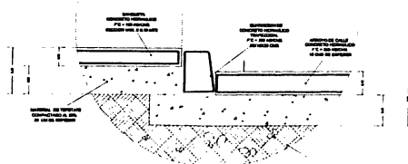
Detalle (C) sección de banqueta
