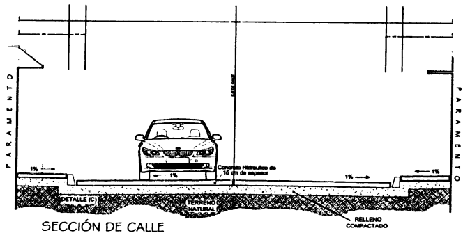
SECCIÓN DE CALLE SIN ESCALA
