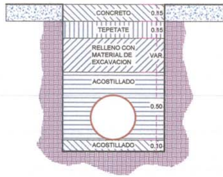
DETALLE ZANJA
