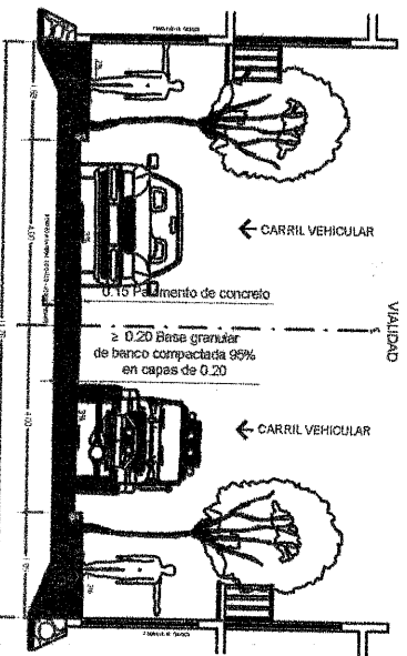
SECCIÓN X-X'
