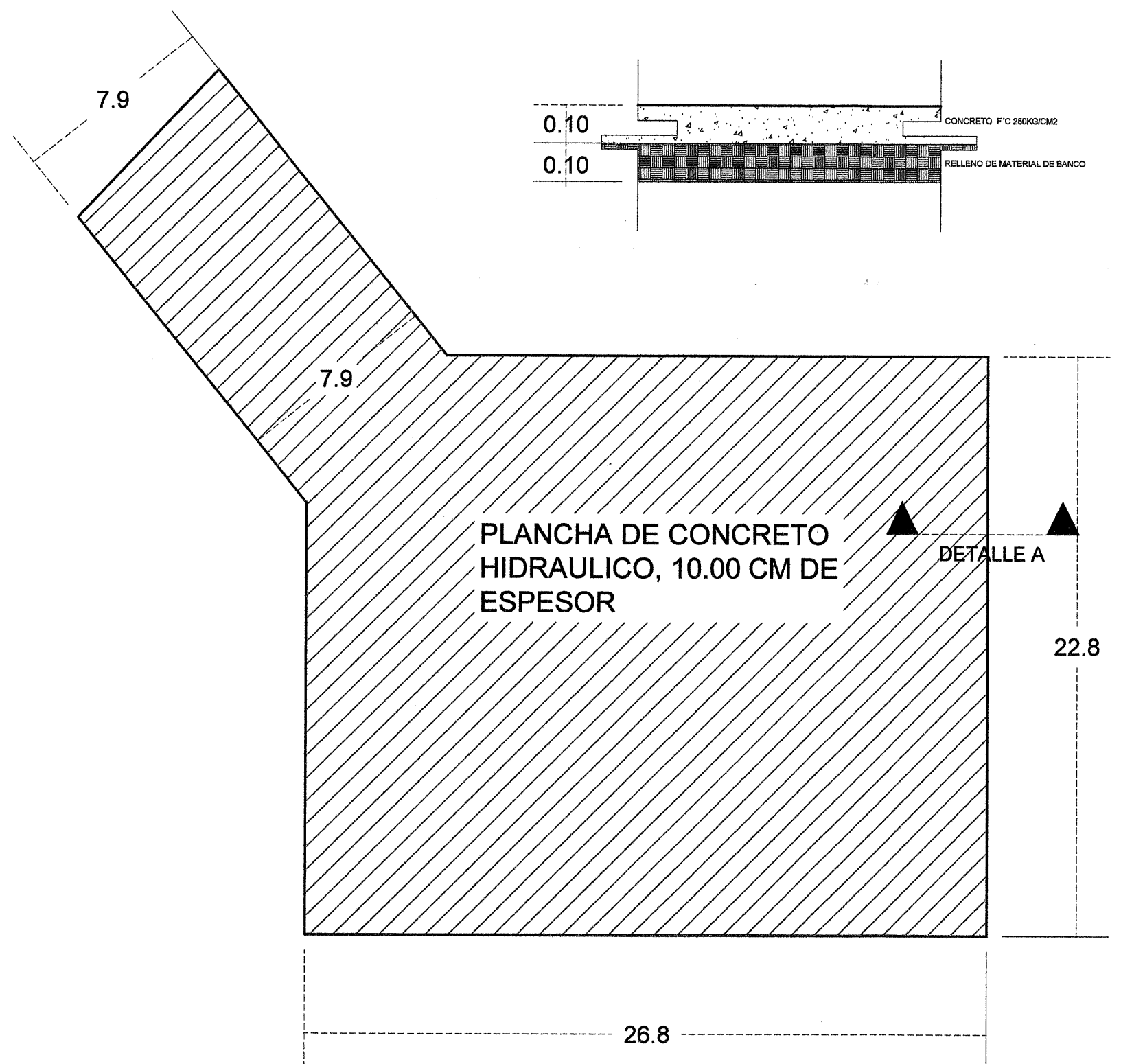
DETALLE A
