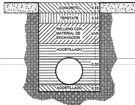
DETALLE ZANJA
