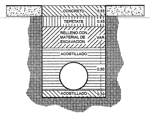
DETALLE ZANJA
