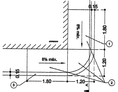
DETALLE RAMPAS
